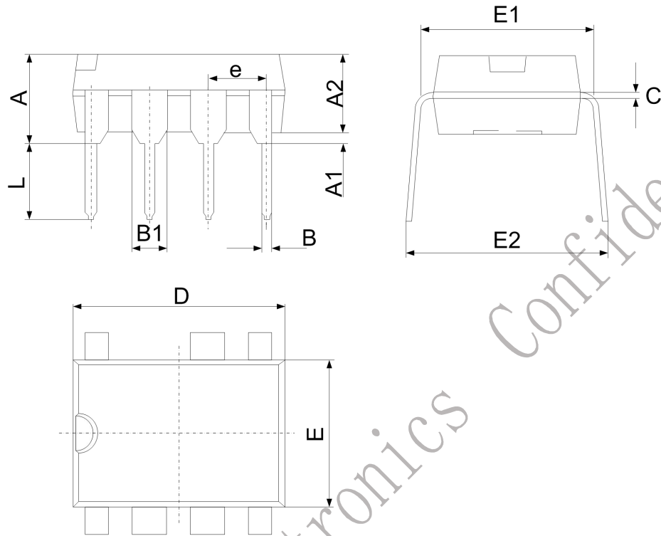
DIP-7
