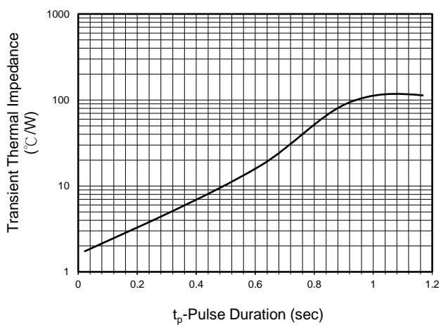
Fig. 5 - Typ. Transient Thermal Impedance
