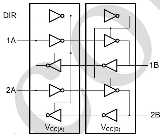
图 2 逻辑框图
