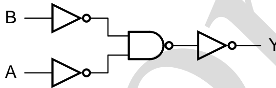
图 3 逻辑框图
