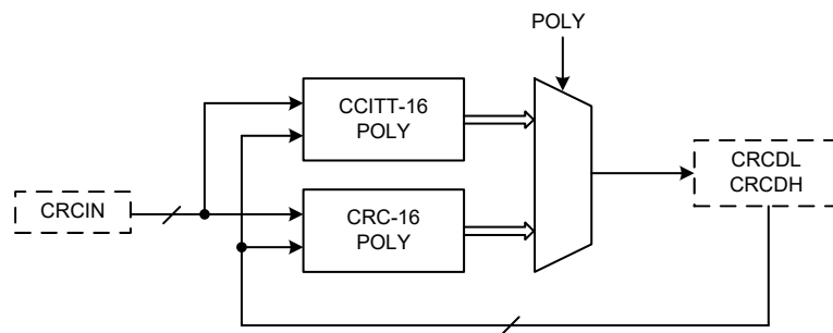
CRC 方框图
