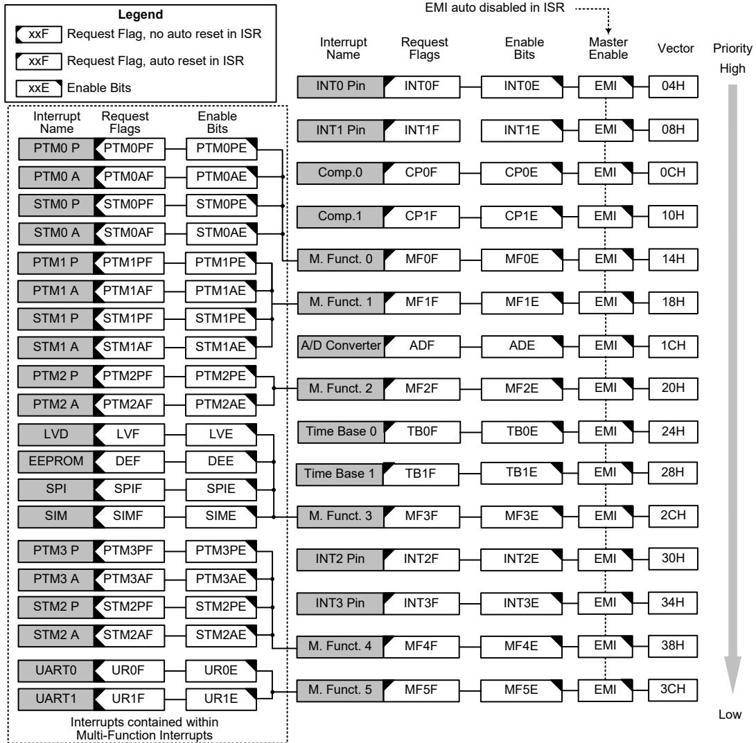
中断结构
