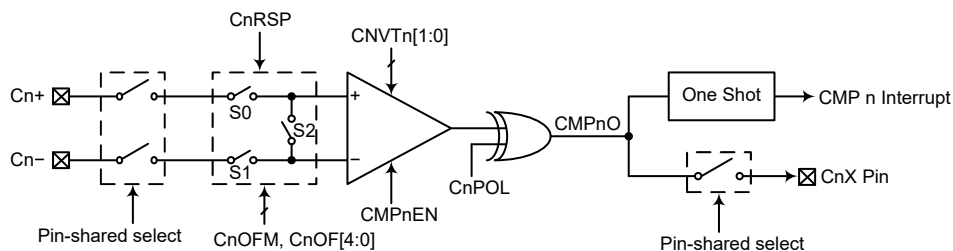
比较器 (n=0~1)
