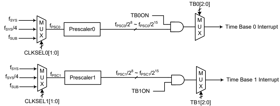
时基中断
