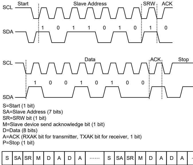
I 2 C 通信时序图
