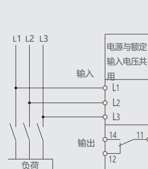
NJB1-X1继电器的接线图
