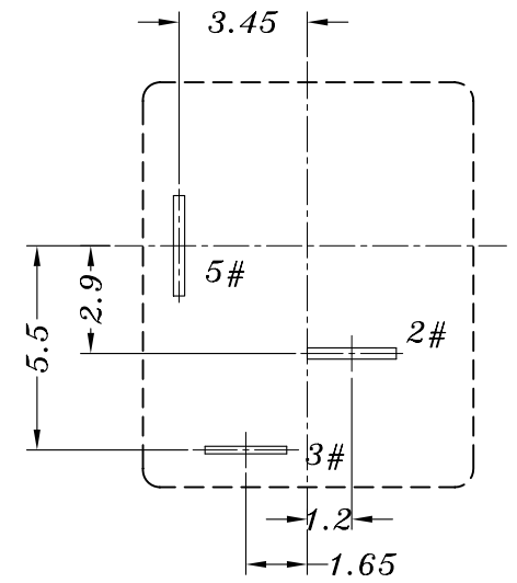
P.C.B LAYOUT
