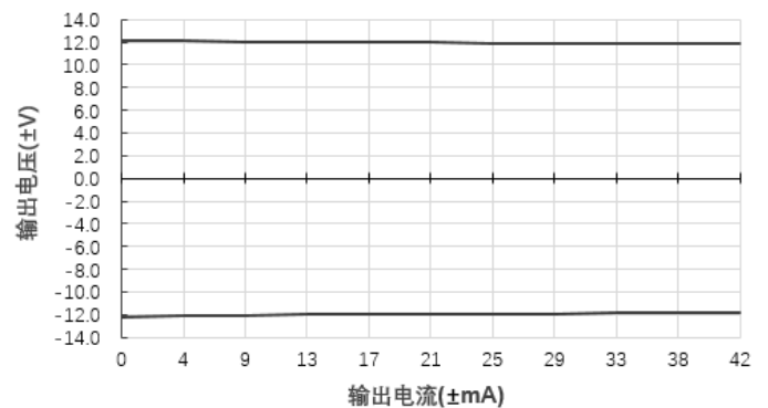
输出电压Vs输出电流(Vin=12V)@E2412S-1WR2
