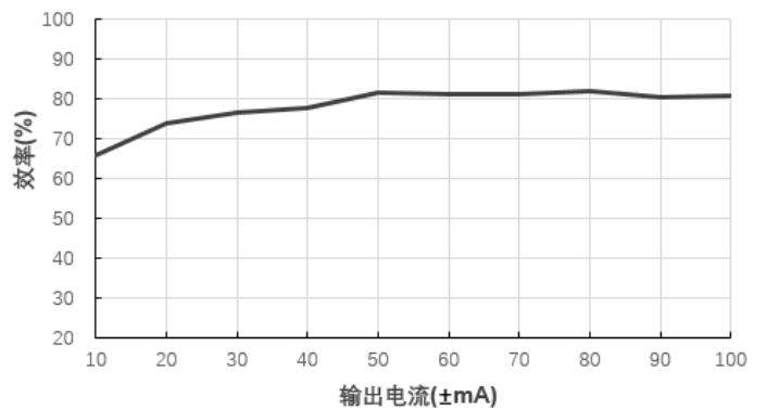
效率Vs输出电流(Vin=12V)@E1205S-1WR2
