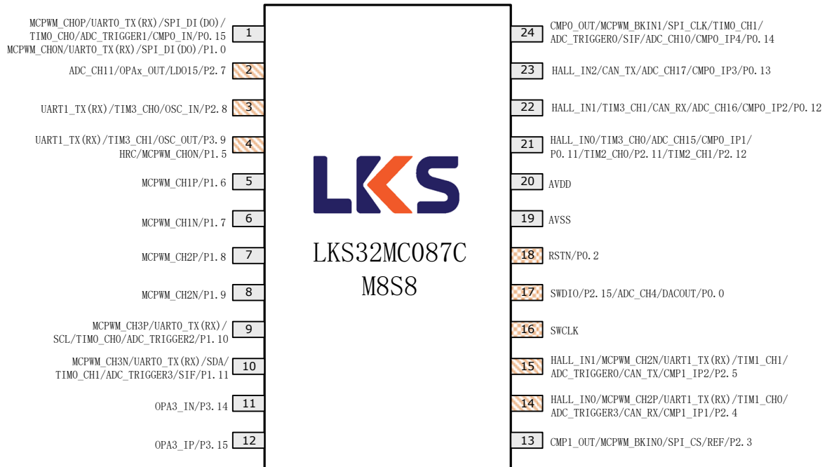
图 3-8 LKS32MC087CM8S8 管脚分布图
