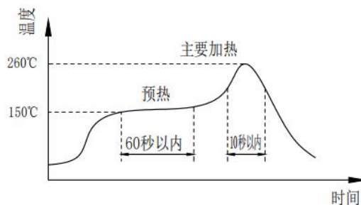
图 3. 回流焊接
