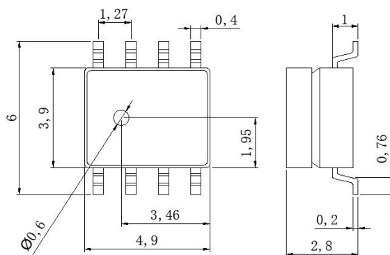
图 1. 外形结构
