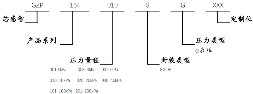
图 2. 选型指南
