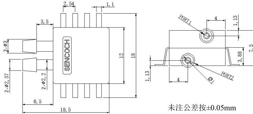
图 1. 外形结构
