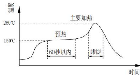
图 3. 回流焊接
