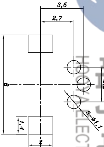
安装尺寸图
