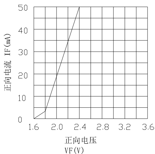
正向电流与正向电压
