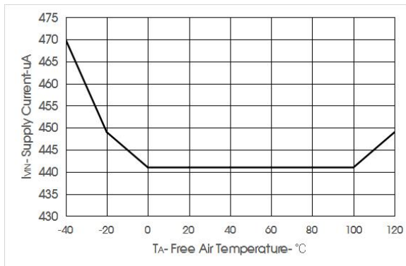
图 1 VIN 平均供应电流 VS 环境温度
