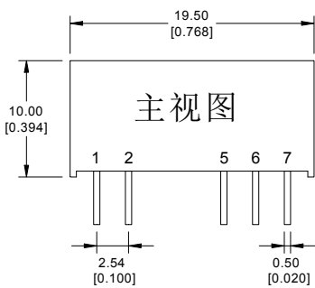
封装尺寸图
