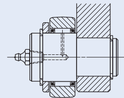
图3 无内圈轴承的安装例
