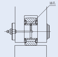
图2 油孔位置和负载方向
