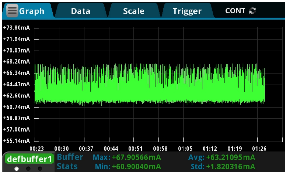
图 8 待机功耗图
