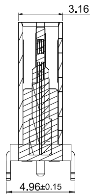
截面 1-1
