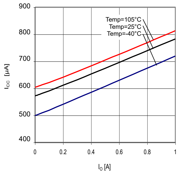
Fig.30 I_o - I_{cc}
