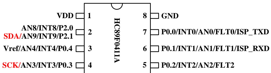
Figure 1-5 SOP8 引脚配置图
