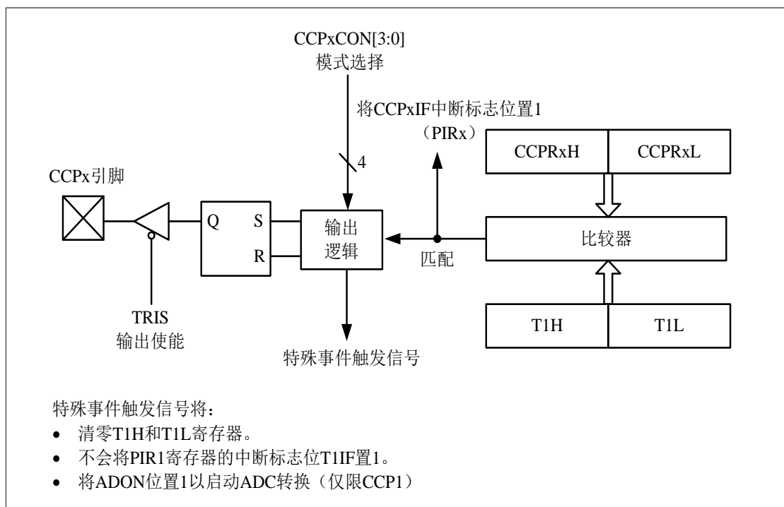
图8-6 比较模式工作原理图
