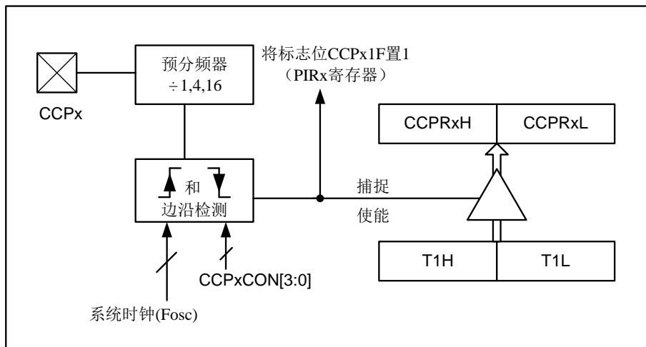
图8-5捕捉模式工作原理图
