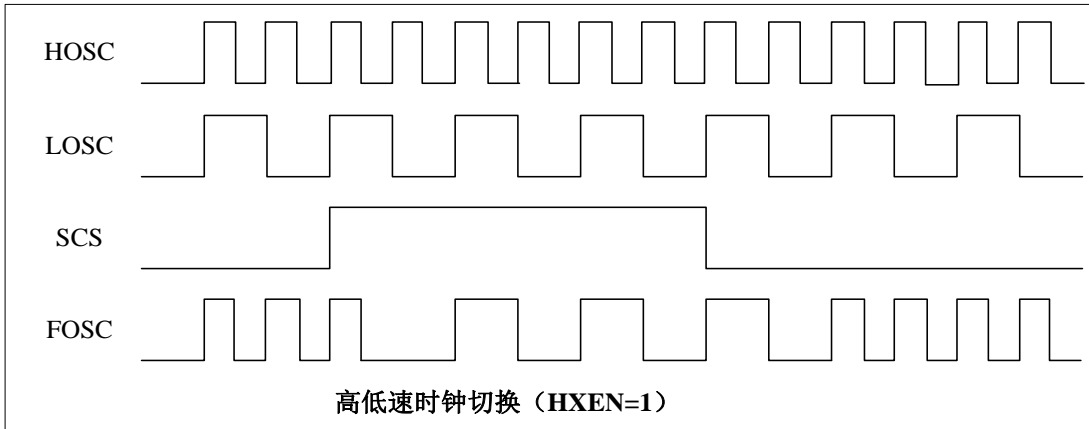
图5-3 高低频切换时序图二
