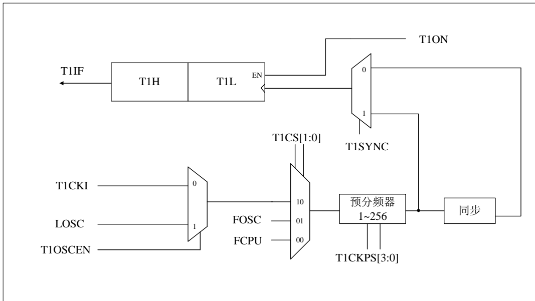
图8-3Timer1模块框图
