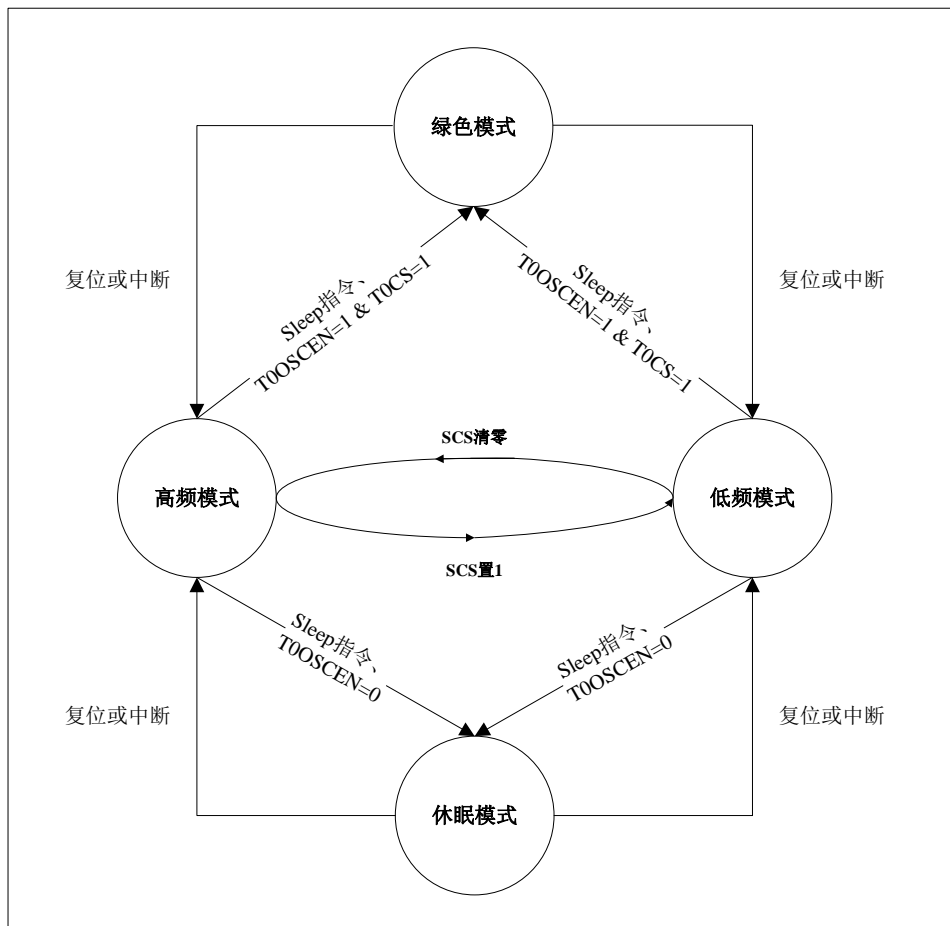
图5-1 系统工作模式转换：
