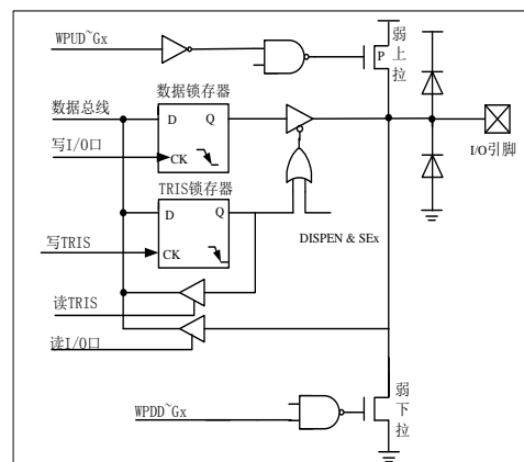
图 1-6: PORTF 口的等效电路
