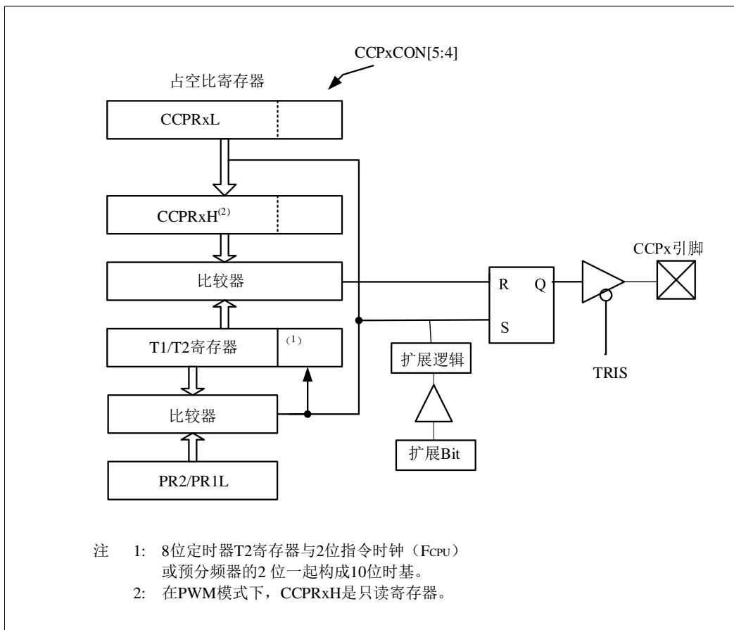
图8-7 PWM模式工作原理图
