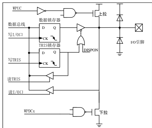
图 1-5: PORTC0 口的等效电路
