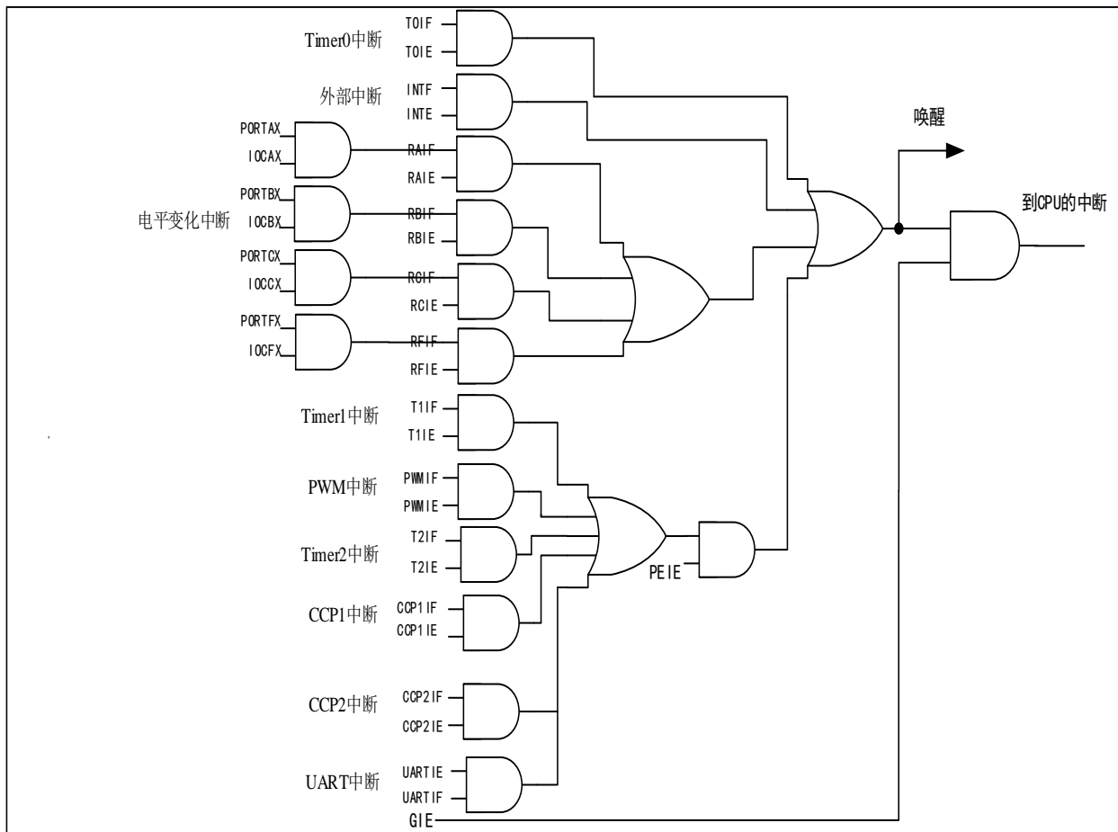
图6-1 中断示意图
