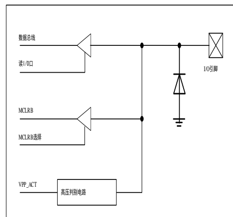
图 1-6: PORTF 口的等效电路
