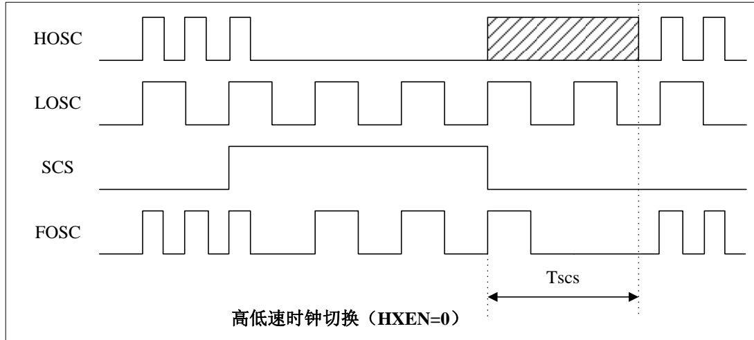
图5-2 高低频切换时序图一
