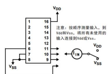
Fig. 4 输入电流
