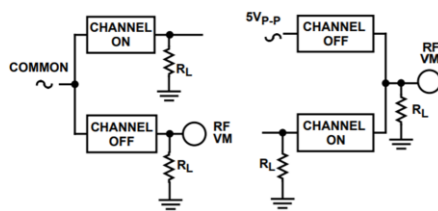
Fig. 9 同一通道信号串扰
