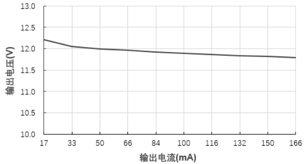
输出电压Vs输出电流(Vin=24V)@B2412S-2WR2
