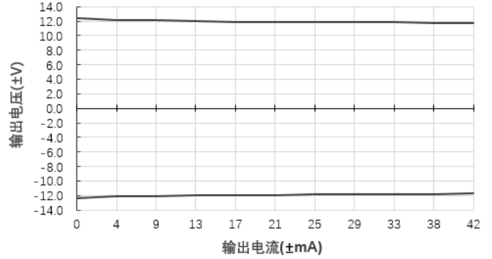
输出电压Vs输出电流(Vin=5V)@A0512S-1WR3
