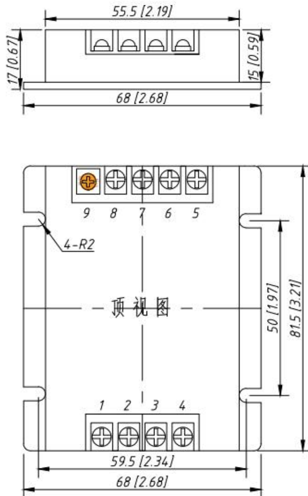
外形尺寸 81.5x68x17mm
