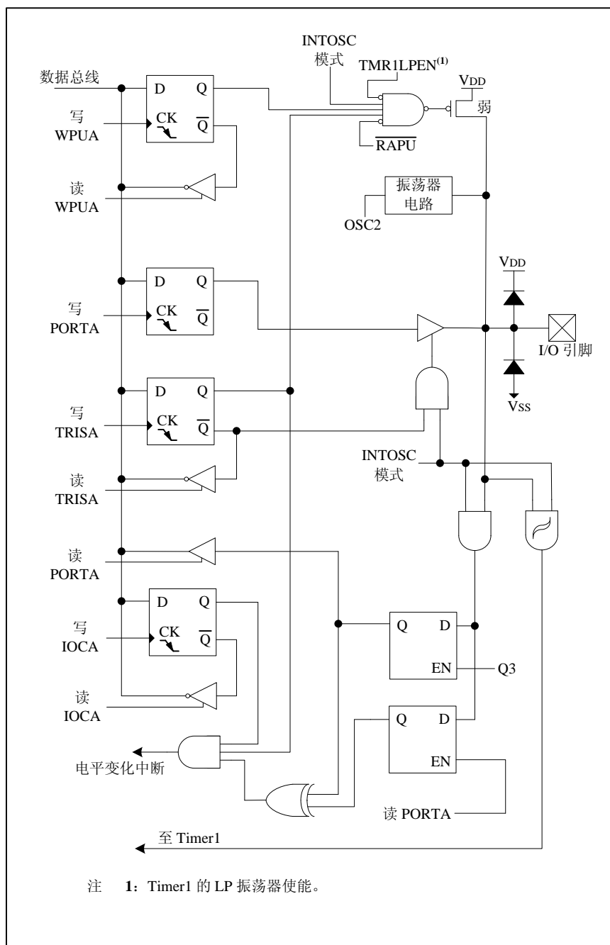
图 6-4-6: PA5 框图
