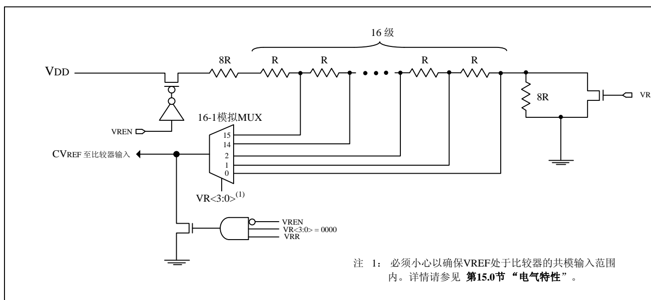
图 10-10-4: 比较参考电压框图
