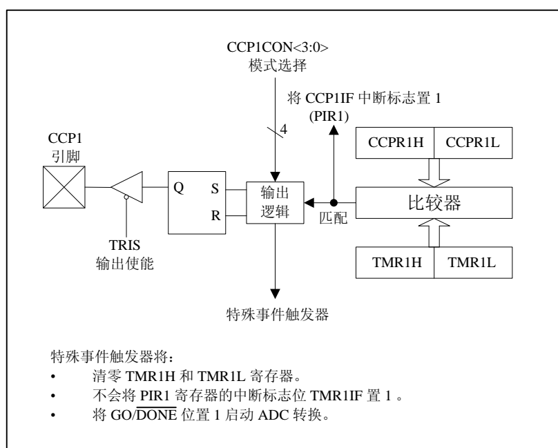
图 8-4-1: 比较模式的工作框图
