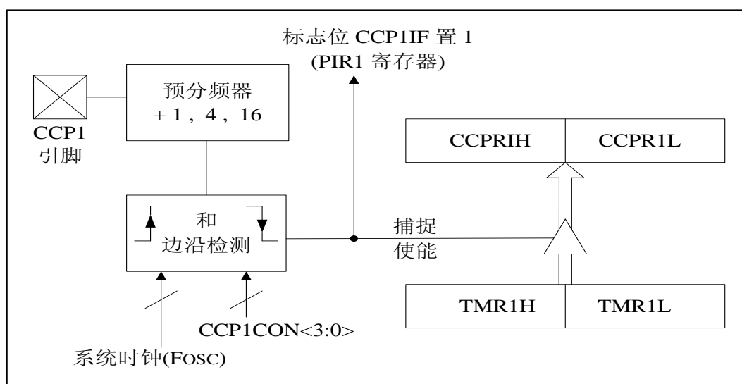
图 8-3-1: 捕捉模式工作原理框图
