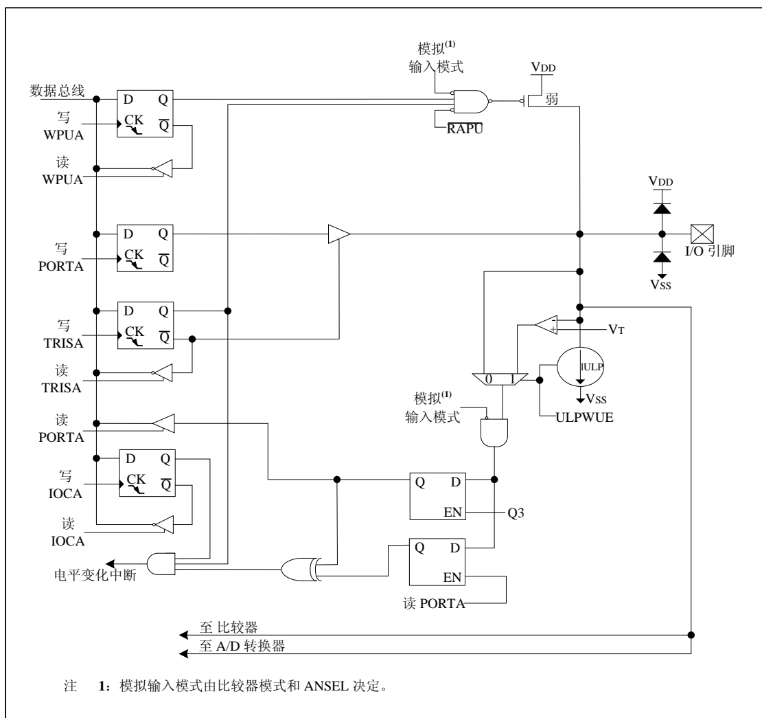
图 6-4-1: PA0 框图
