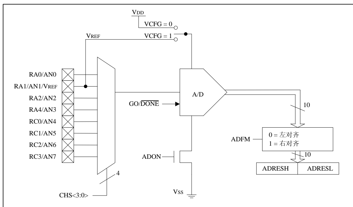
图 9-1：ADC 框图
