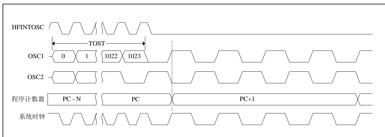
图 4-7-3: 双速启动
