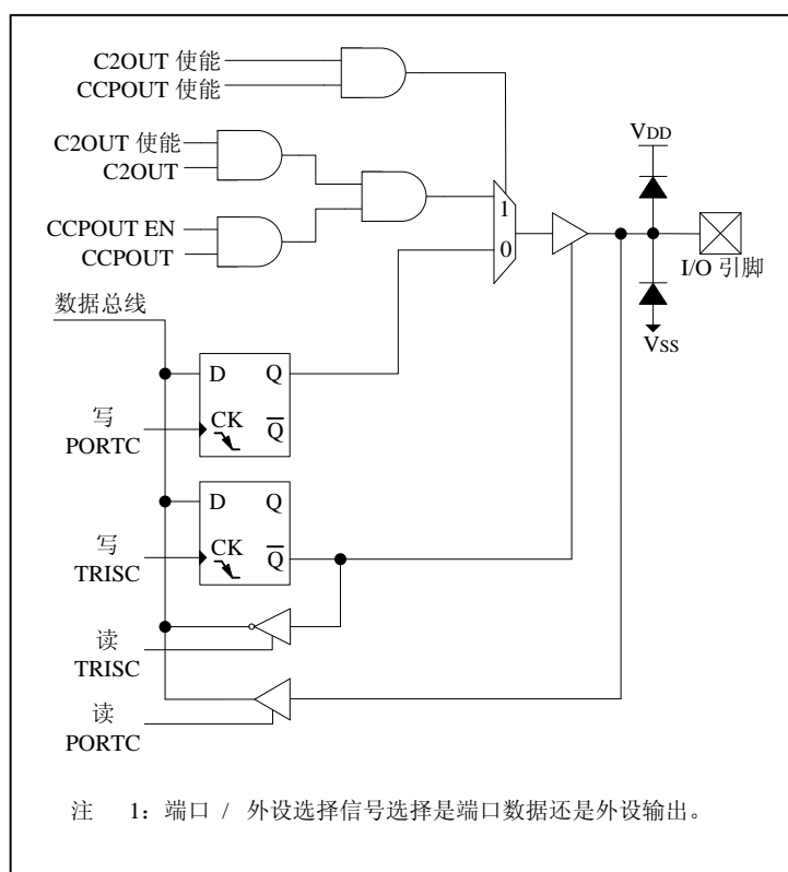
图 6-5-5: PC4 框图
