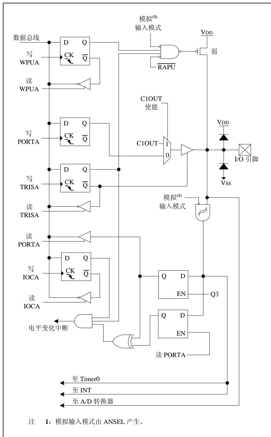
图 6-4-3: PA2 框图
