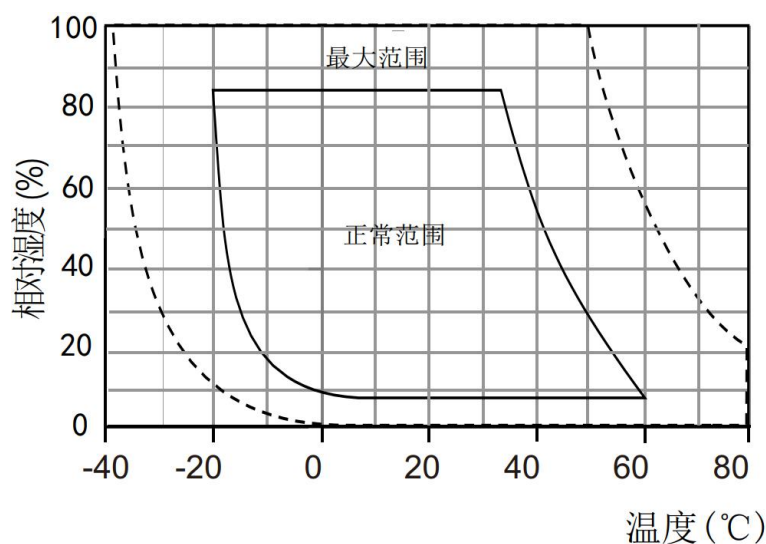
图4 工作条件
