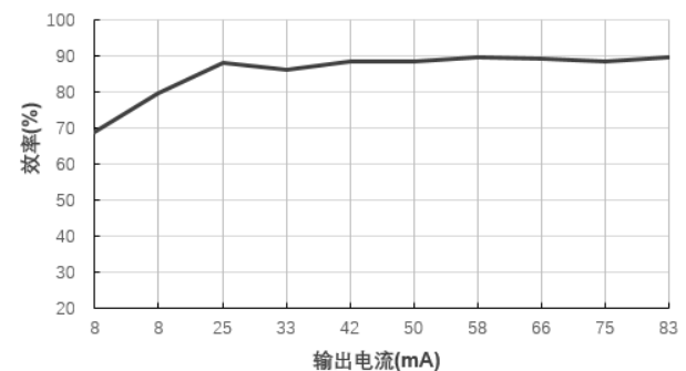
效率Vs输出电流(Vin=12V)@F1224S-2WR2
