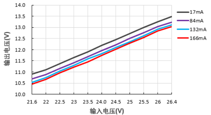
输出电压Vs输入电压@F2412S-2WR2
