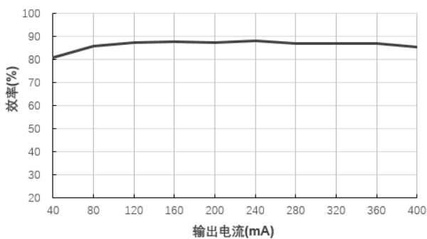
效率Vs输出电流(Vin=12V)@F1205S-2WR2
