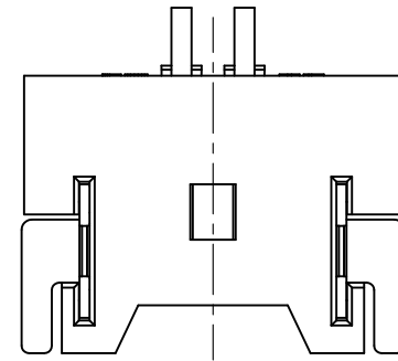
2~3 Pin结构外形(锁扣窗口)
