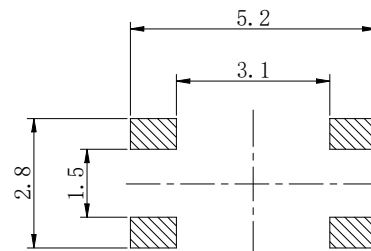
焊接尺寸图
