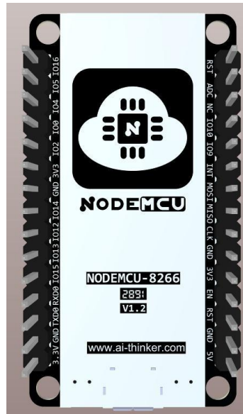
NodeMCU-8266 管脚示意图
