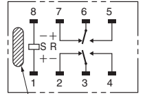
端子配置/内部连接图 (BOTTOM VIEW)
