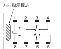
端子配置/内部连接图 (BOTTOM VIEW)
