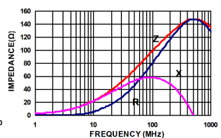
FBC1608-101Y
