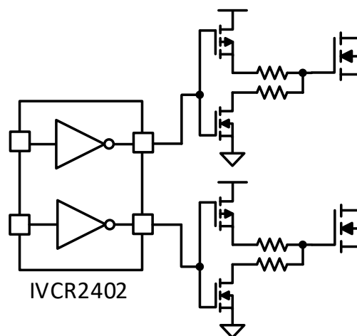
图 8. 两通道分别驱动
