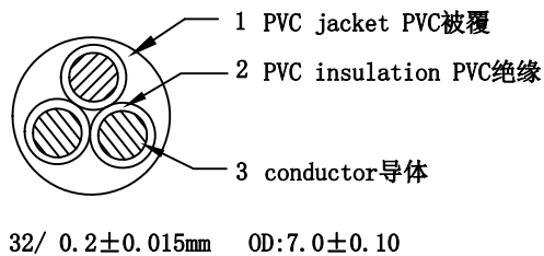
线材截面图:
