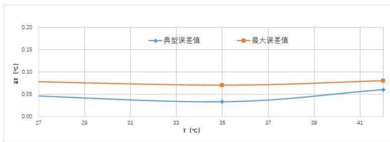
图 7- 1 MTS01 精度误差曲线
