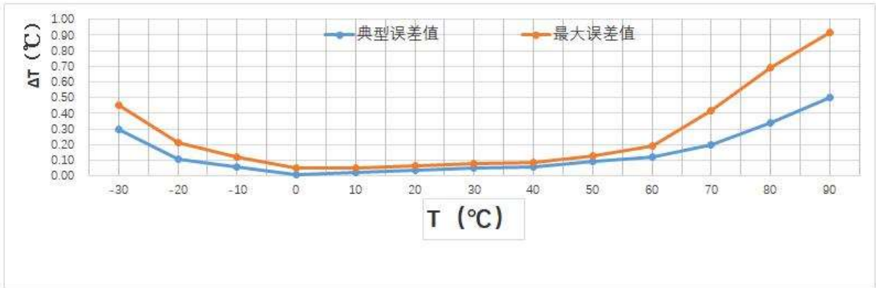
图 7- 2 MTS01Z 精度误差曲线
