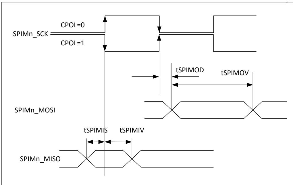
图 4-24 SPI-Mn 接口时序图 (CPHA=0)
