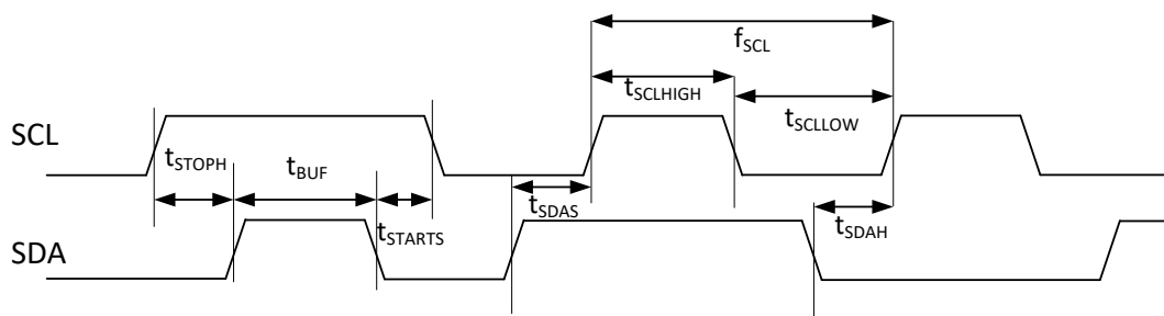
图 4-29 I2C 接口时序图
