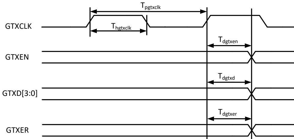
图 4-18 GMII 模式发送接口时序图
