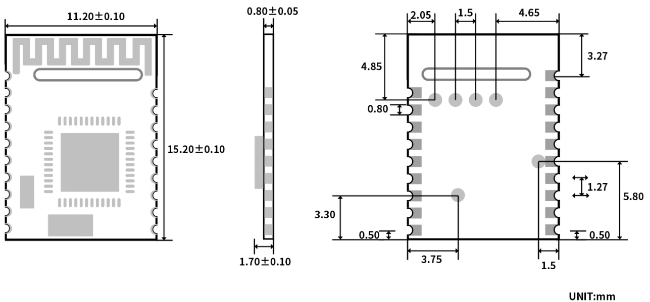
图 2. RF-BM-ND08C 尺寸图
