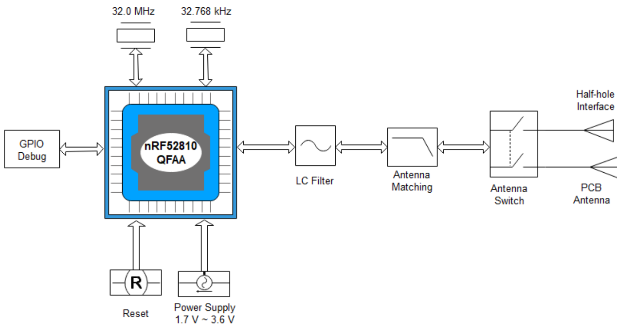
图 1. RF-BM-ND08C 原理框图
