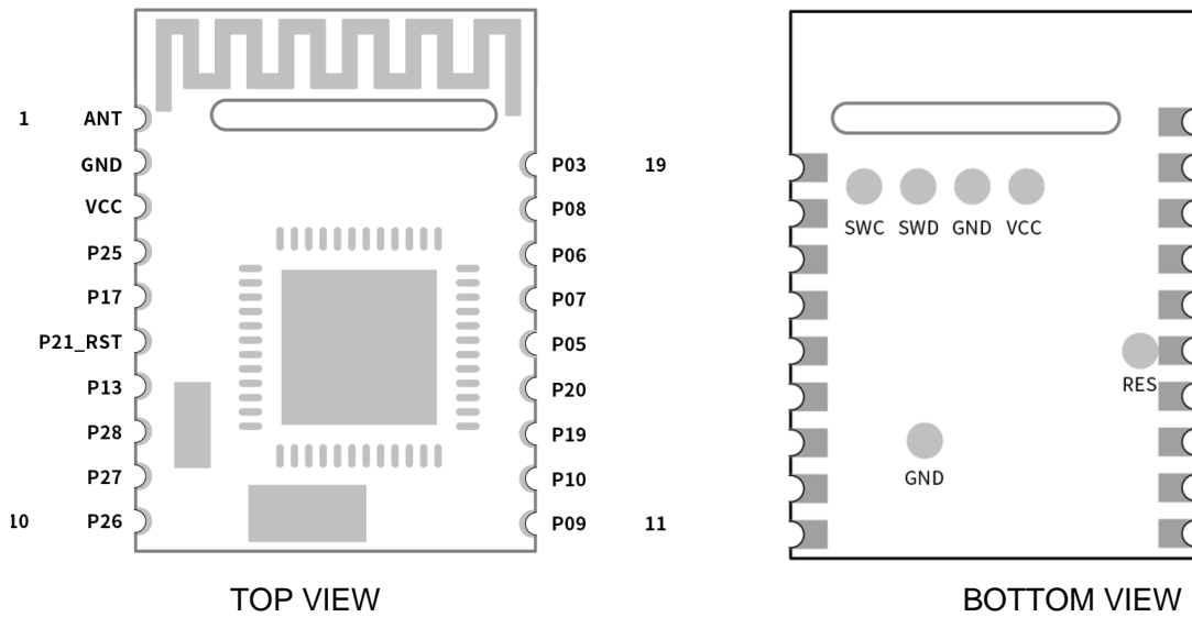
图 3. RF-BM-ND08C 引脚图
