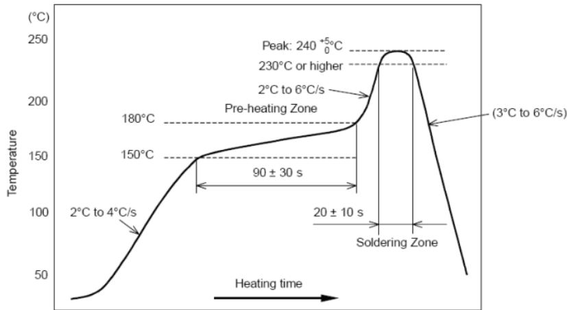
图 6. 部件的焊接耐热性温度曲线(焊接点)
