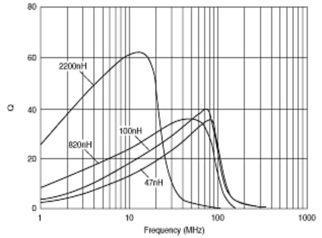
Q频率特性
