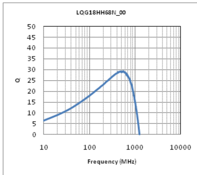
Q频率特性
