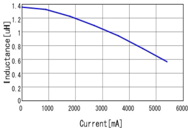
L-Current特性
