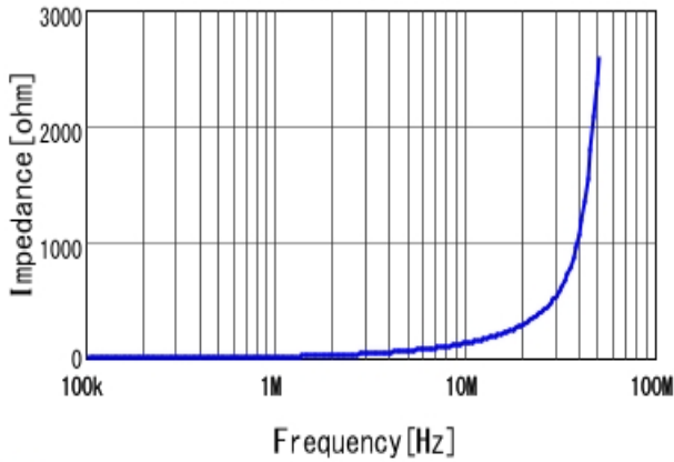
■ 1277AS-H-2R2M |Z|
