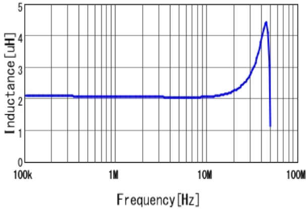
■ 1277AS-H-2R2M L
