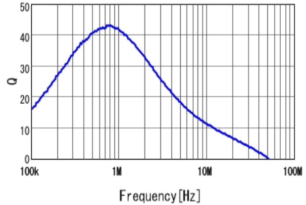
■ 1277AS-H-2R2M Q
