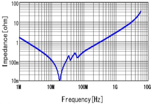
■ GRM3195C1H104GA05 |Z| DC0V, 25degC
