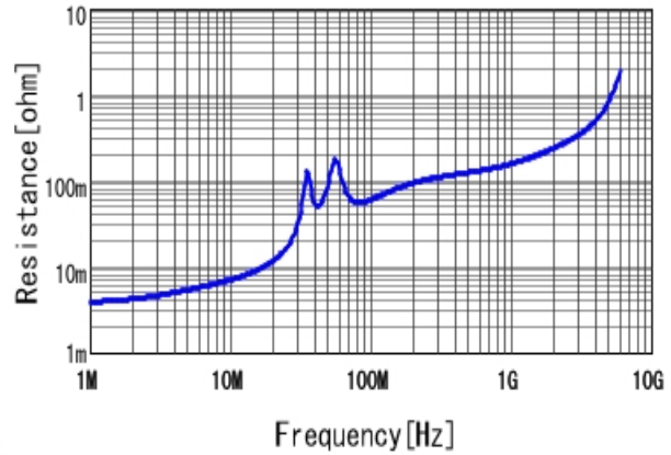
■ GRM3195C1H104GA05 R DC0V, 25degC
