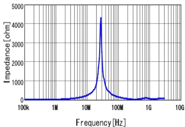
■ FDVE0630-H-3R3M |Z|
