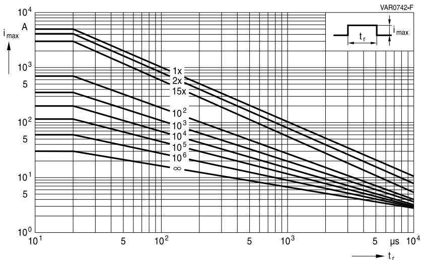
SIOV-SNF14K350 ... K625E2S5K1
