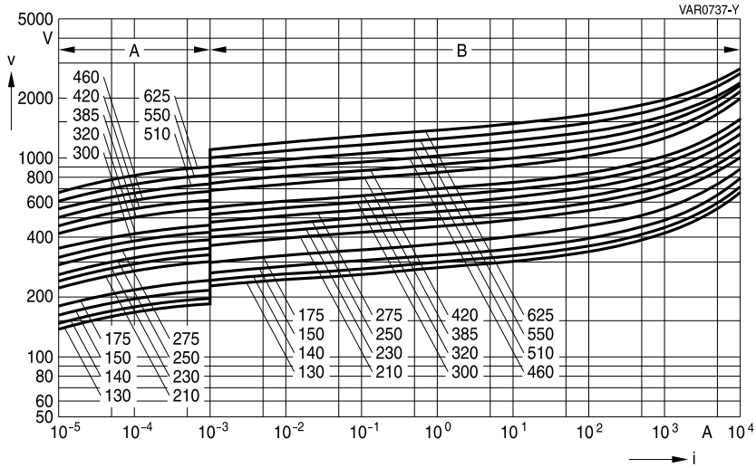
SIOV-SNF20 ...
