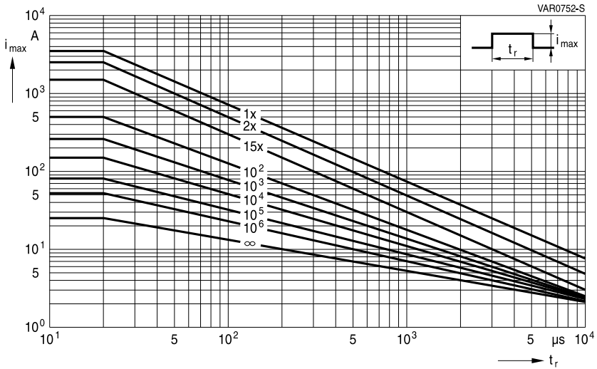
SIOV-SNF10K130 ... K320E2S5K1
