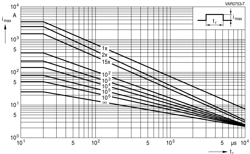
SIOV-SNF10K350 ... K625E2S5K1
