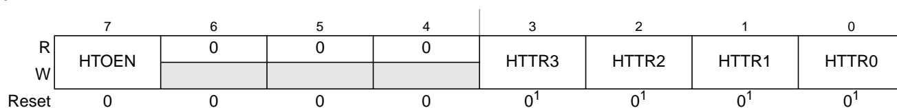
Figure 3-8. VREGHTTR
