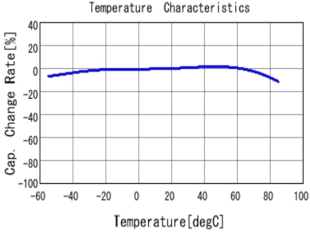
■ GRM188R60G226MEA0 C-Temp. capchange, DCO. 0V, ACO. 2V rm
