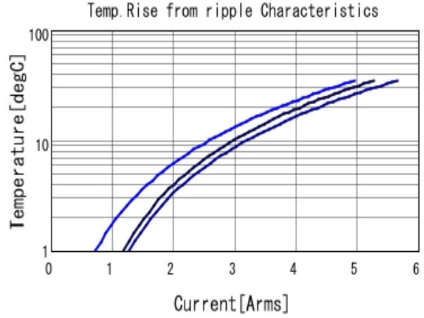
GRM188R60G226MEA0 Temp. rise ■ 80kHz ■ 400kHz ■ 800kHz
