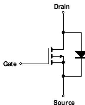
P-Channel MOSFET
